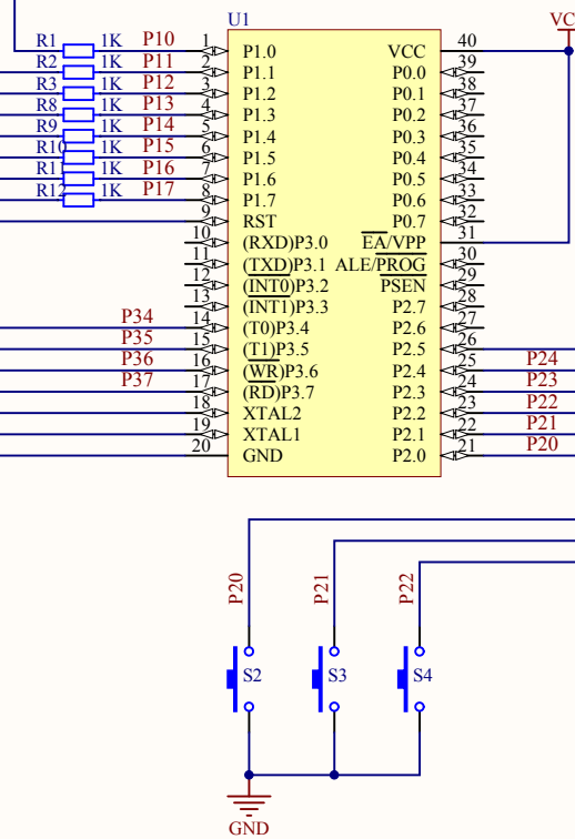
按键电路
