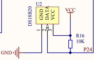
18b20温度传感器
